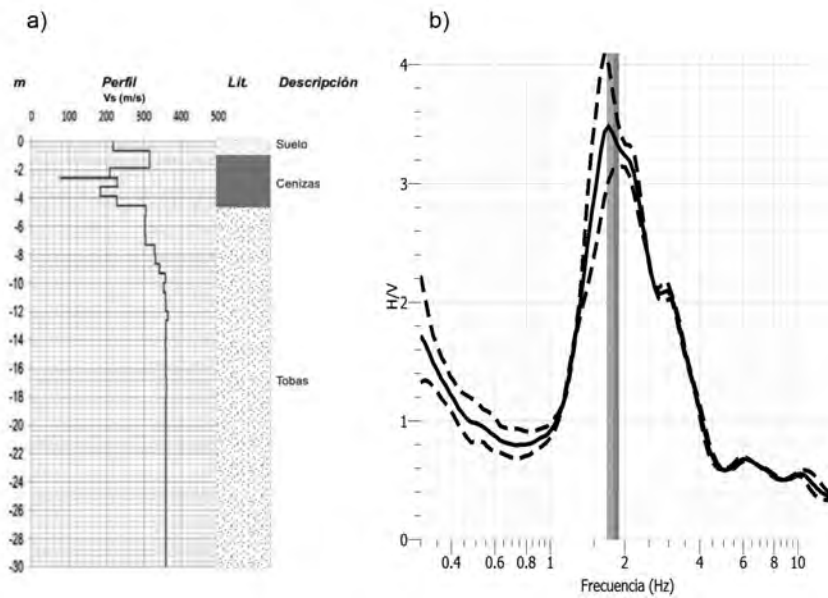
Figura 7. Alajuela Centro: (a) Perfil de suelos en el sitio (Vargas, 2010). (b) Razón espectral H/V.
