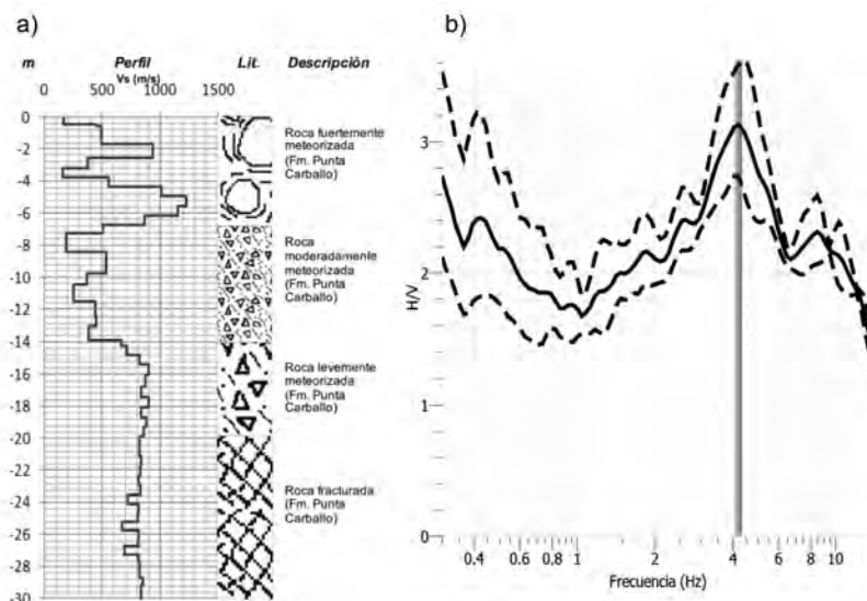
Figura 2. Cerro Chiqueros: (a) Perfil de suelos en el sitio (Vargas, 2010). (b) Razón espectral H/V.
