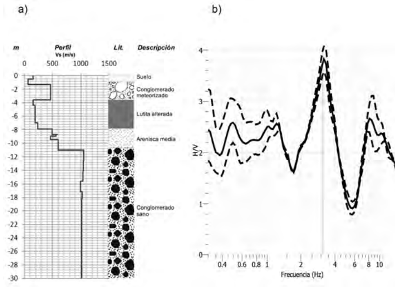
Figura 6. Naciente, Santa Ana: (a) Perfil de suelos en el sitio (Vargas, 2010). (b) Razón espectral H/V.
