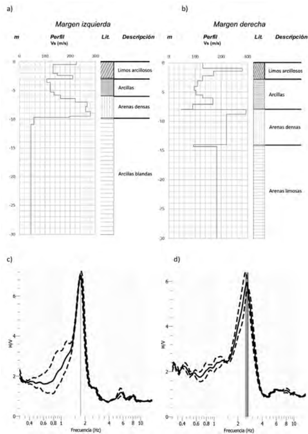
Figura 10. Río Purires, Tobosí, Cartago: (a) Perfil de suelos en el sitio, margen izquierda (Coto & Vargas, 2010). (b) Perfil de suelos en el sitio, margen derecha (Coto & Vargas, 2010). (c) Razón espectral H/V, margen izquierda. (d) Razón espectral H/V, margen derecha.
