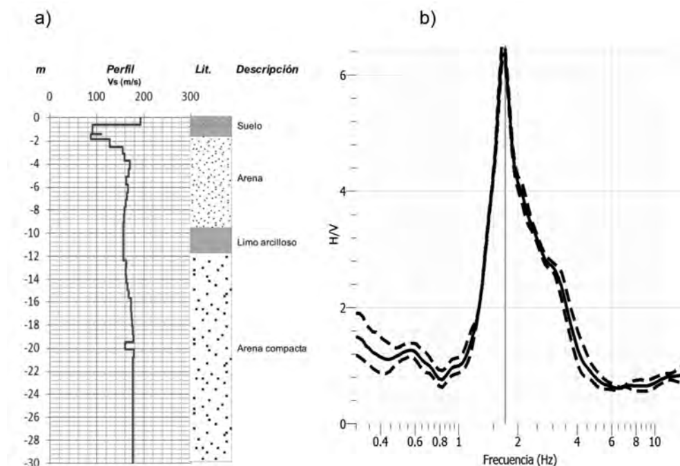
Figura 5. Bulevar, Jacó: (a) Perfil de suelos en el sitio (Vargas, 2010). (b) Razón espectral H/V.
