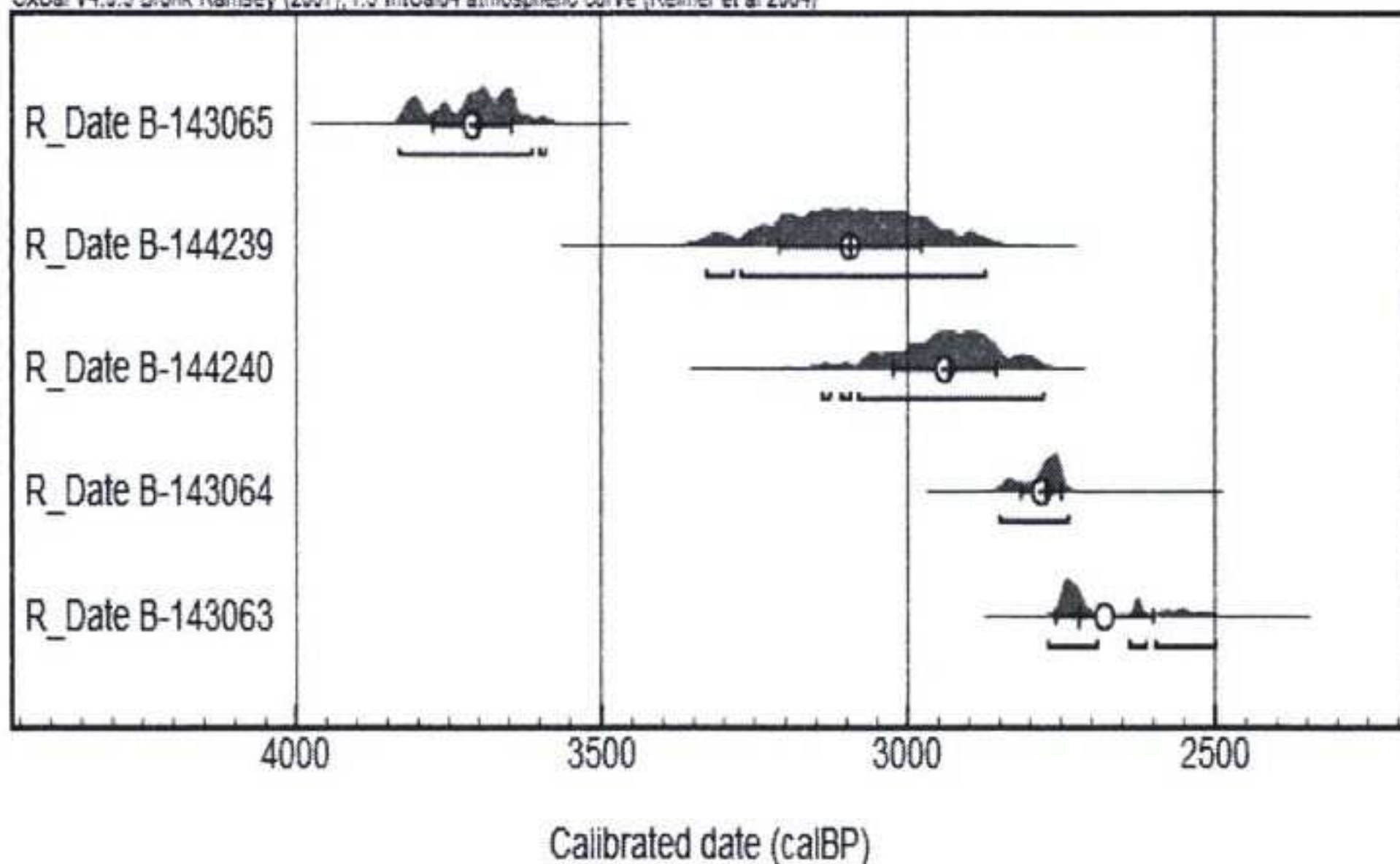
Figura 4. Probabilidad estadística de fechas radiométricas (2- \sigma ) cal. A.P.: Raphia taedigera : \beta -143065, estrato II; \beta -144239, estrato III; \beta -144240 estrato II; Elaeis oleifera : \beta -143064, estrato II/III; Raphia taedigera : \beta -143063, estrato II.
