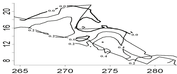
Figura 4c. Patrón espacial de correlaciones para el tercer modo de la temperatura superficial del aire. El contorno más grueso es el de cero correlación.
