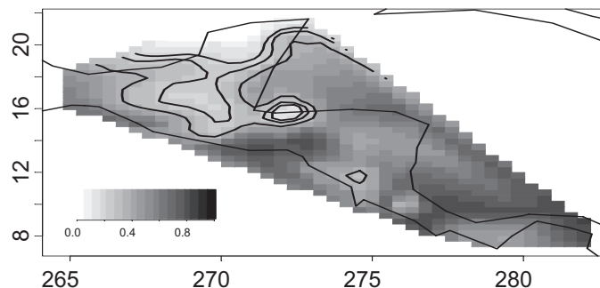
Figura 5. Patrón espacial de la habilidad estadística predictiva del campo de la temperatura superficial del aire en Centroamérica para la predicción del trimestre de mar-abr-may usando la temperatura superficial del mar en dic-ene-feb como predictor. Los valores se calcularon como la correlación entre las series de tiempo observadas y las predichas por el modelo del análisis de correlación canónica usando validación cruzada. Los contornos representan los niveles de confianza del 90, 95 y 99 por ciento en orden creciente.
