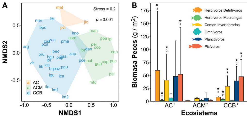
Fig. 4. A. NMDS de la composición de la comunidad de peces en los tres tipos de ecosistemas coralinos: (AC) arrecifes de coral vivos, (ACM) arrecifes de coral muertos, y (CCB) comunidades coralinas sobre basaltos. B. Biomasa promedio (+ IC 95%) de peces según su grupo alimenticio estimada para los tres tipos de ecosistemas arrecifales. Los asteriscos (*) indican diferencias significativas ( P < 0.005 ) entre ecosistemas arrecifales específicos. / Fig. 4. A. NMDS of fish community composition in the three types of coral ecosystems: (AC) living coral reefs, (ACM) dead coral reefs, and (CCB) coral communities on basalts. B. Average biomass (+ 95% CI) of fish by food group estimated for the three reef ecosystem types. Asterisks (*) indicate significant differences ( P < 0.005 ) between specific reef ecosystems.
