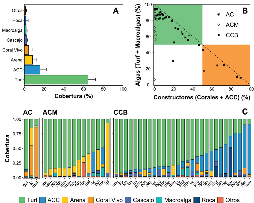
Fig. 2. A. Cobertura del fondo promedio (+ IC 95 %) de los sitios arrecifales visitados. ACC: algas coralinas costrosas. B. Relación entre la cobertura de constructores (corales y ACC) y algas (turf + macroalgas). C. Cobertura del fondo para cada uno de los sitios categorizados como arrecifes de coral vivos (AC), arrecifes de coral muertos (ACM) y comunidades coralinas sobre basaltos (CCB) visitados. / Fig. 2. A. Average bottom cover (+ 95 % CI) of the reef sites visited. ACC: crustose coralline algae. B. Relationship between builder cover (corals and ACC) and algae (turf + macroalgae). C. Bottom cover for each of the sites categorized as living coral reefs (AC), dead coral reefs (ACM) and coral communities on basalts (CCB) visited.
