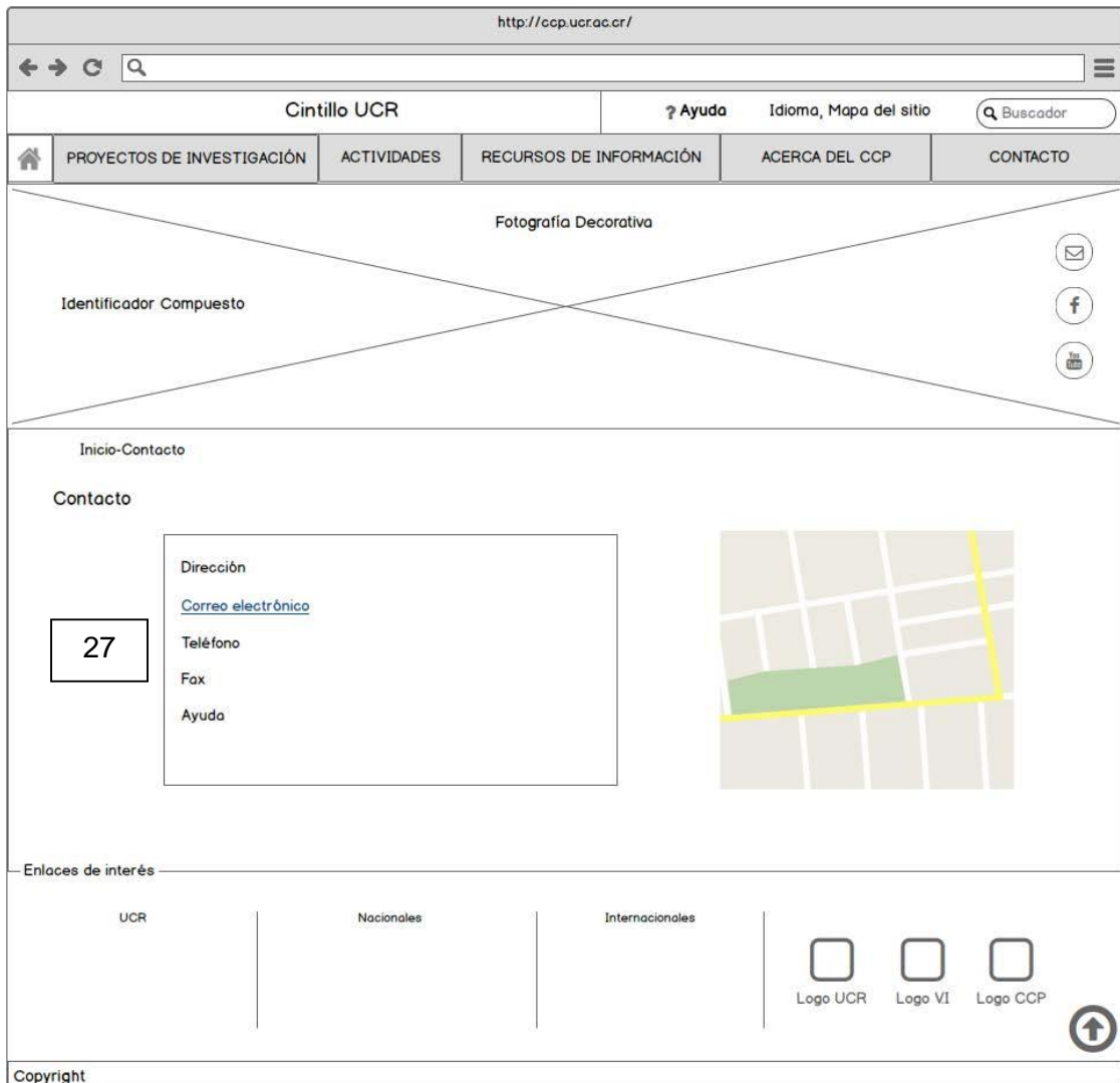
Figura 72: Wireframe Contacto
