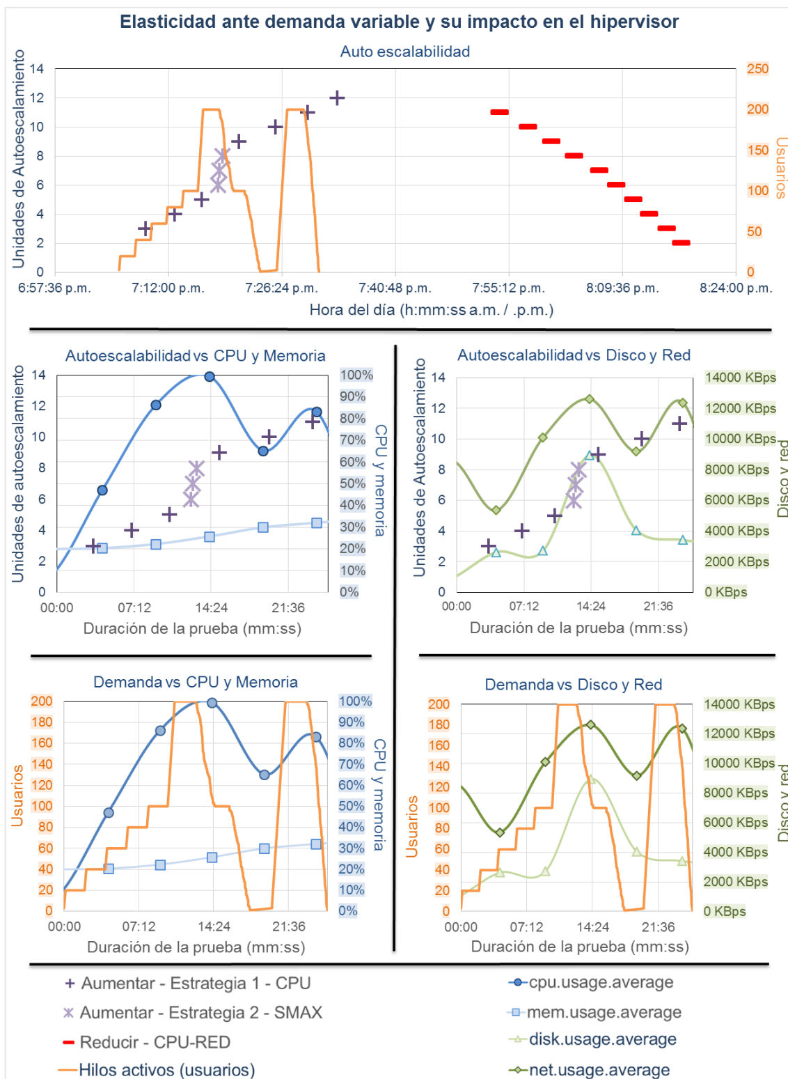
Figura 17. Gráficos de resultados. Elasticidad ante demanda variable y su impacto en el hipervisor durante la prueba de auto escalabilidad
