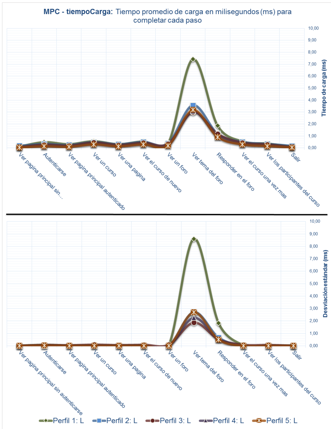
Figura 22. Gráfico de resultados. Tiempo de carga en las pruebas de rendimiento según la herramienta MPC
