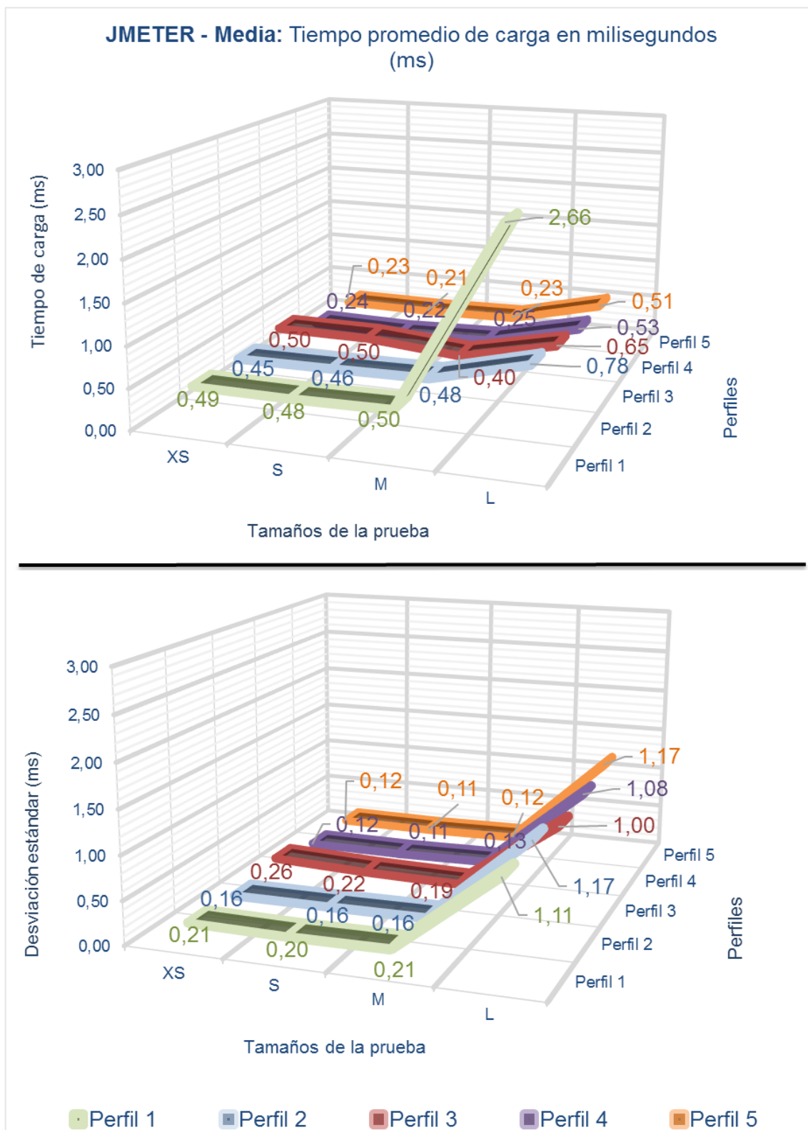
Figura 18. Gráfico de resultados. Tiempo promedio de las pruebas de rendimiento según JMETER
