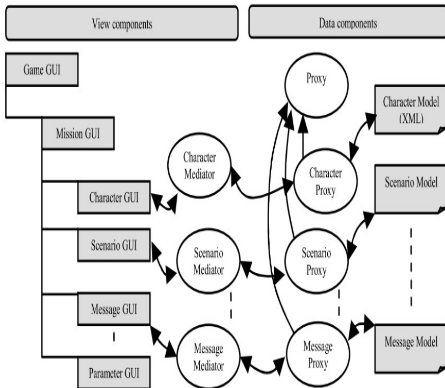
Figura 7.23 Arquitectura SeGAE
