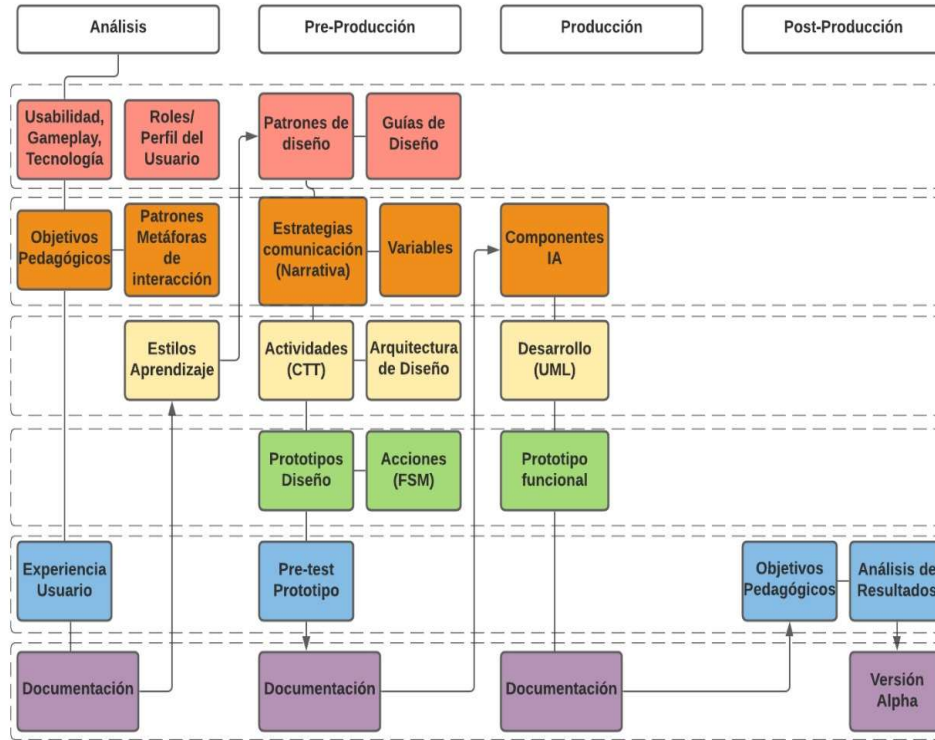
Figura 6.9 Metodología MECONESIS
