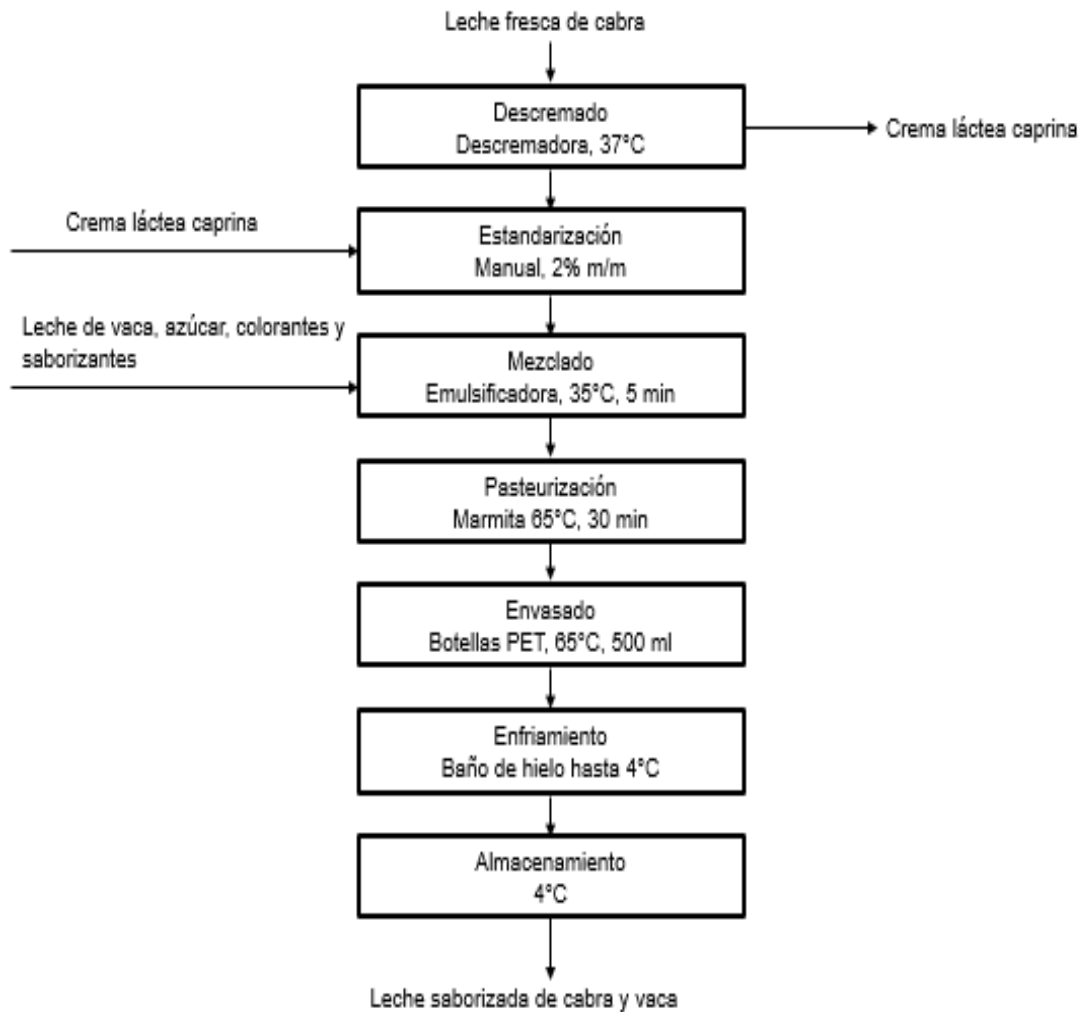
Figura 4.3.1.1. Diagrama de flujo para la elaboración de leches saborizadas a partir de leche de vaca y cabra (Adaptado de: Hui, 2006; Silverson, s.f).
