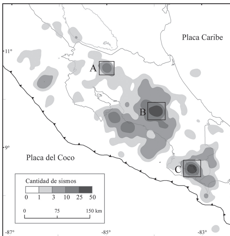
Fig. 5: Cantidad de sismos por área calculada en celdas cuadradas de 100 km 2 . El volcán Tenorio (A), el área entre Cartago y Tarrazú (B) y el golfo Dulce (C) son las zonas que presentaron la mayor cantidad de sismos localizados durante el 2018.
