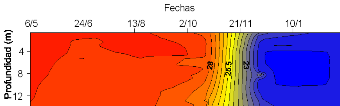
Figura 7. Contorno de temperatura ( ^{\circ}\text{C} ) en el Sitio 1, Bahía Salinas, Guanacaste.
