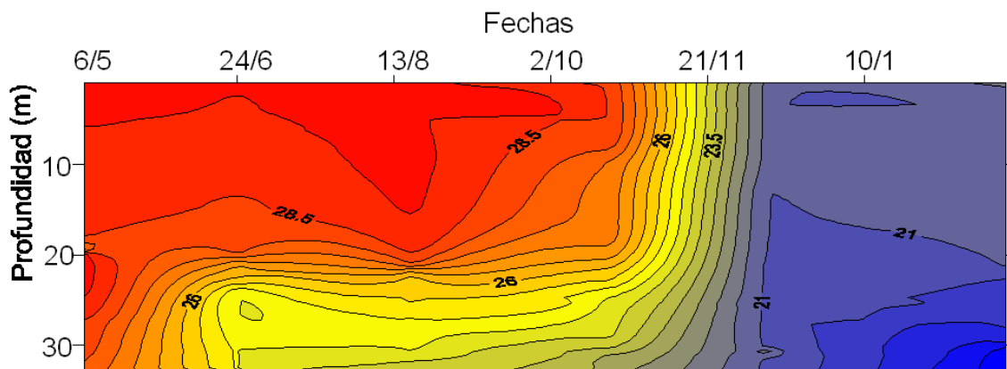
Figura 9. Temperatura ( ^{\circ}\text{C} ) en el Sitio 2, Bahía Salinas Guanacaste.
