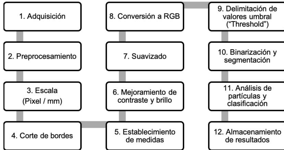
Figura 3 Proceso del análisis digital de imágenes utilizado para evaluar los granos de arroz ( Oryza sativa L.). Costa Rica, 2022.
